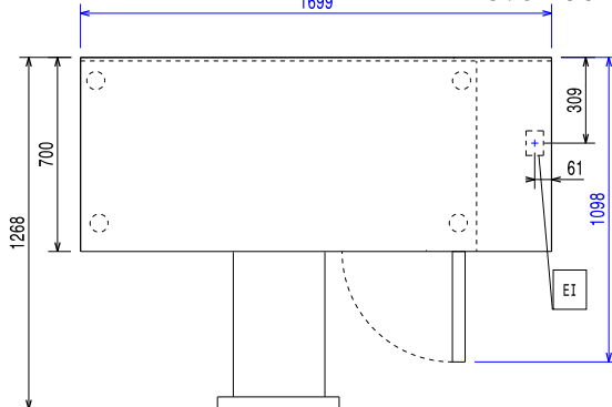
Boven aanzicht
